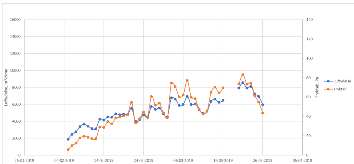
Figur A4. Luftydelsen og tryktab i vinterkampagnen som døgnmiddel. Den 16-03-2019 var der et strømudfald på renseren og perioden indgik derfor ikke i beregningerne.
