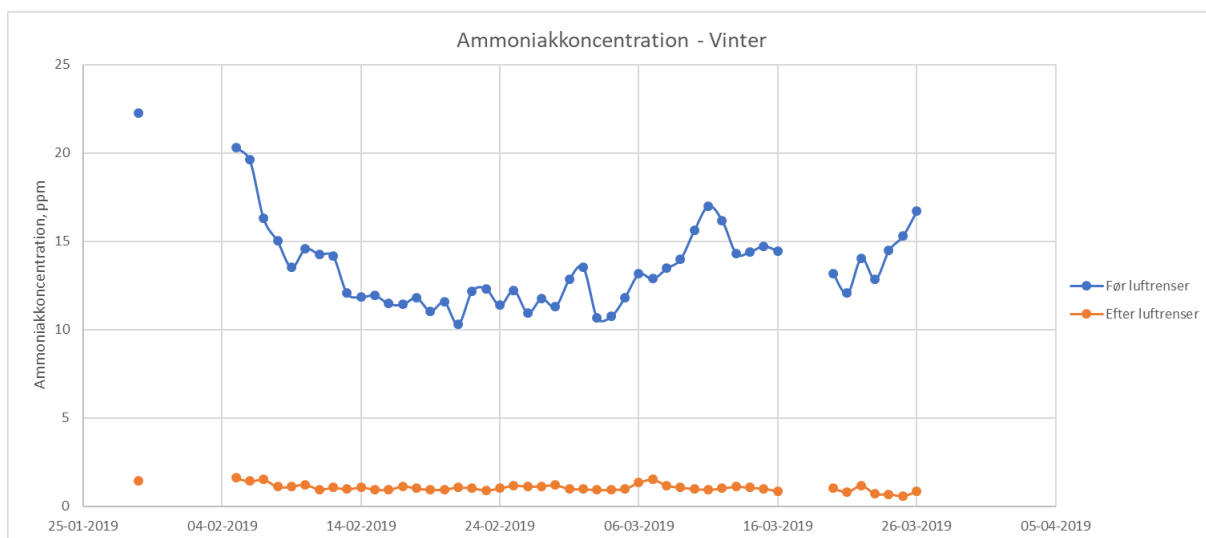
Figur A2. Dagsmiddel af ammoniakkekoncentration før og efter luftreneren i vinterkampagnen. Et strømafbud fra den 16-03-2019 til den 18-03-2019 medførte, at der ikke blev målt med INNOVA. Derudover er perioden fra den 30-01-2019 til den 04-02-2019 ikke medtaget, da kuldioxidkoncentrationen var forskellig før og efter luftreneren.
