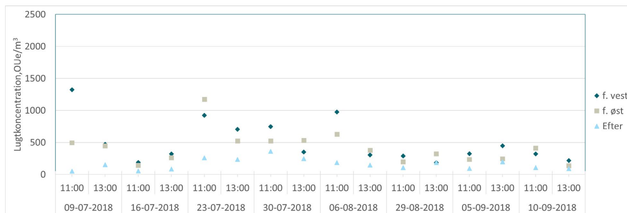
Figur A5. Sommermålinger af lugtkoncentration henholdsvis før og efter luftrensere.
