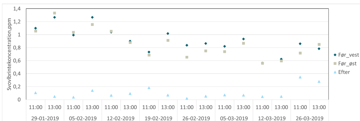
Figur A8. Gennemsnitlig svovlbrintekonzentration på måledage i vinterkampagnen.
